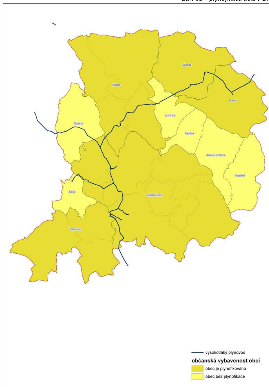
Obr. 11 – plynifikace obcí v ORP Železný Brod
