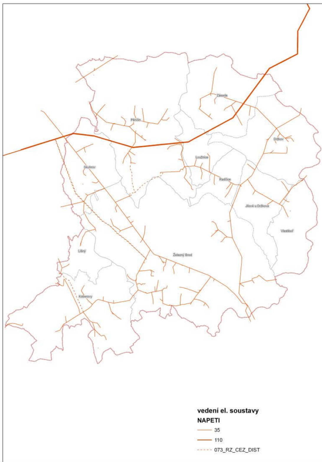
Obr. 14 – elektrosoustava v ORP Železný Brod
