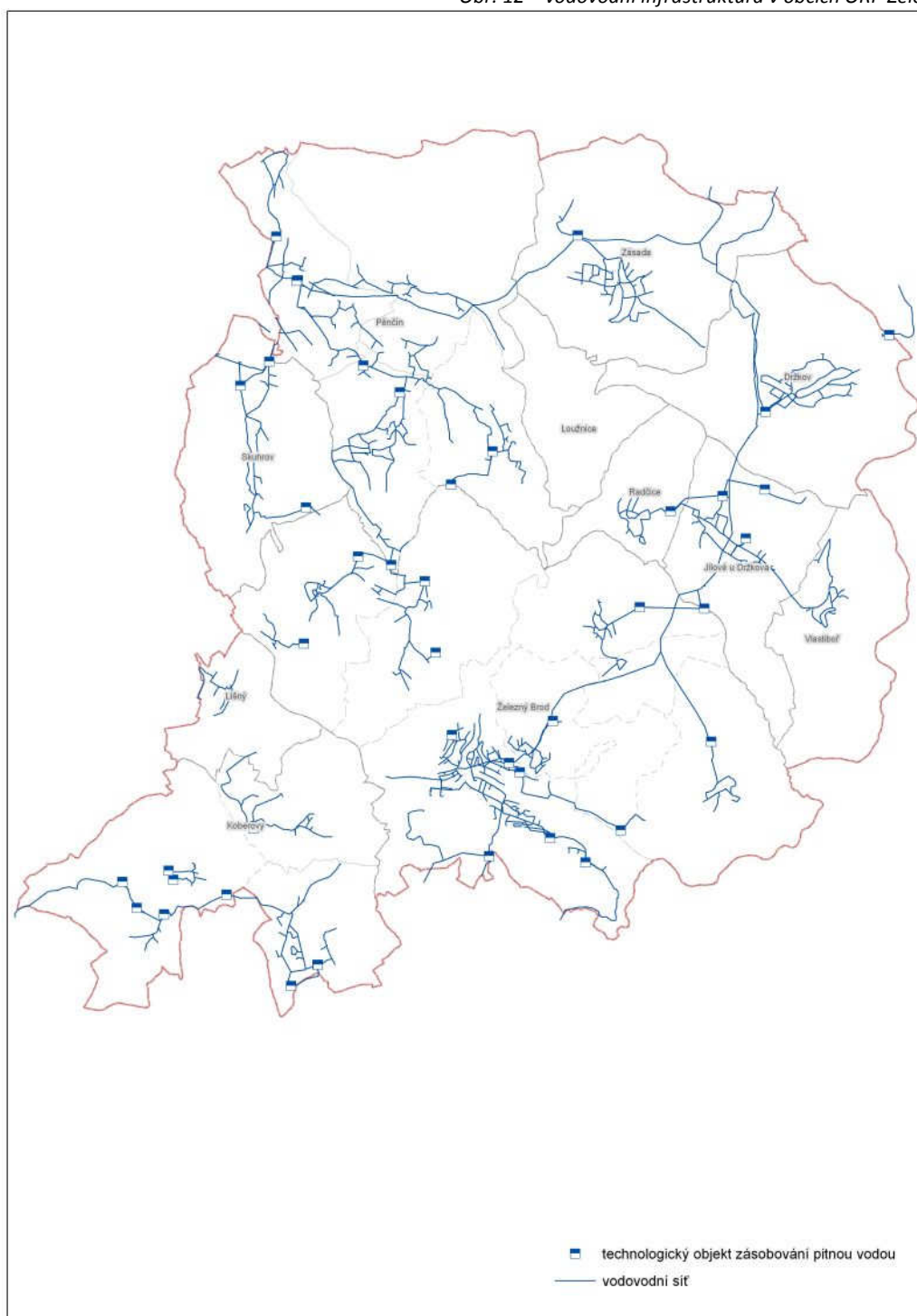
Obr. 12 – vodovodní infrastruktura v obcích ORP Železný Brod
