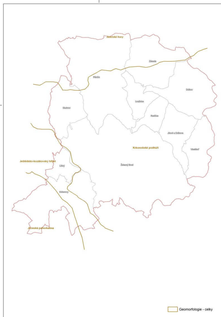
Obr. 4 – geomorfologie - celky
