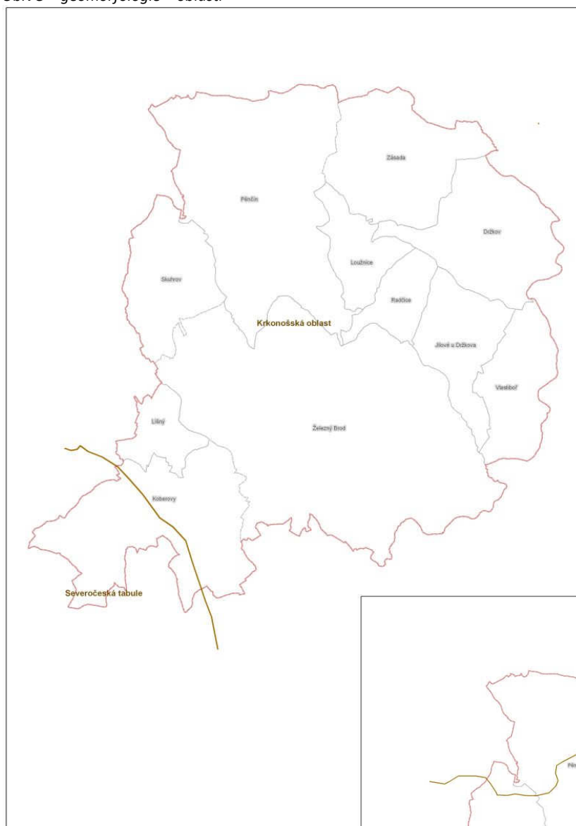
Obr. 3 – geomorfologie – oblasti
