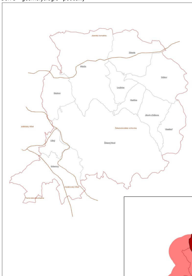
Obr. 5 – geomorfologie - podcelky
