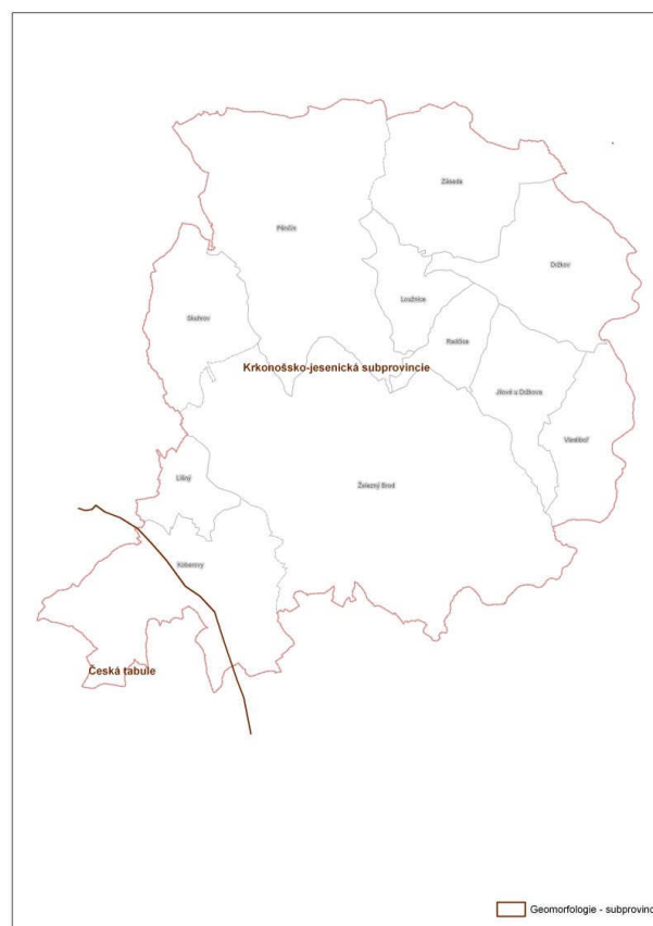
Obr. 2 Geomorfologické subprovincie
